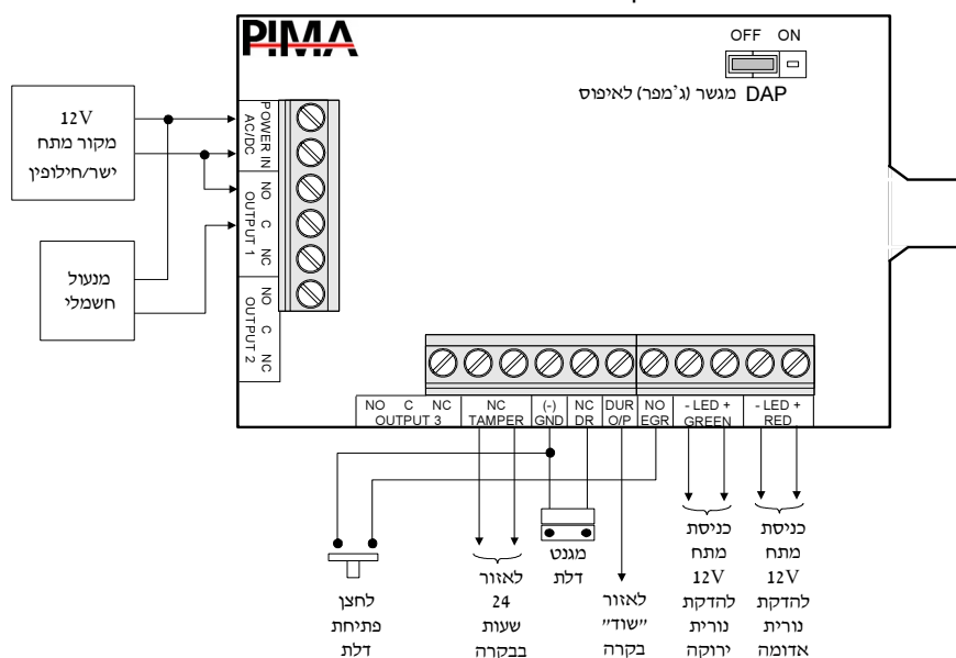
איור 1 – יציאת ממסר ושתי יציאות טרנזיסטור
